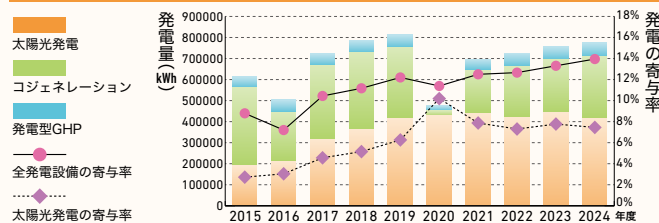
年度毎の発電量
